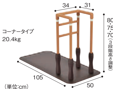
コーナータイプ MNTPCRBR 00054-000132
