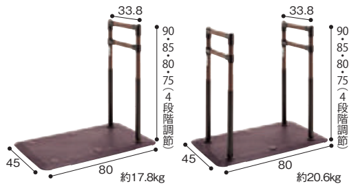
BZK-01 (片手すり) 01265-000248
