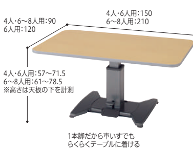
ペダルを踏むだけで昇降やキャスター収納ができる。
